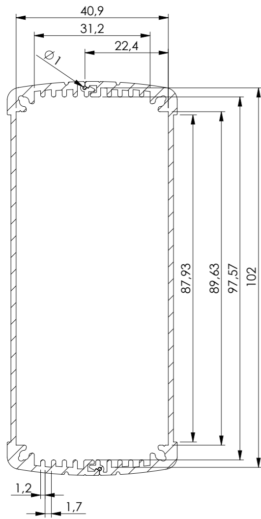
SEZIONE A-A
