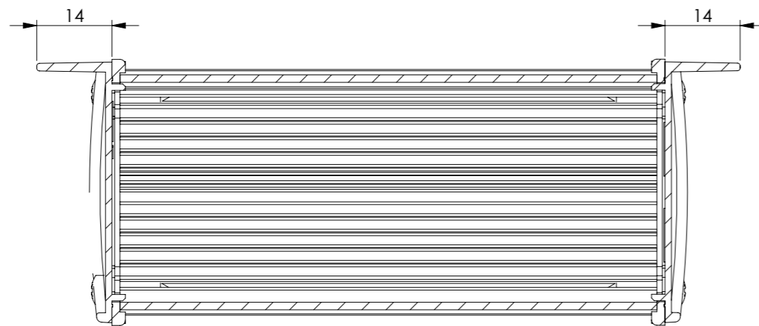
SEZIONE B-B
