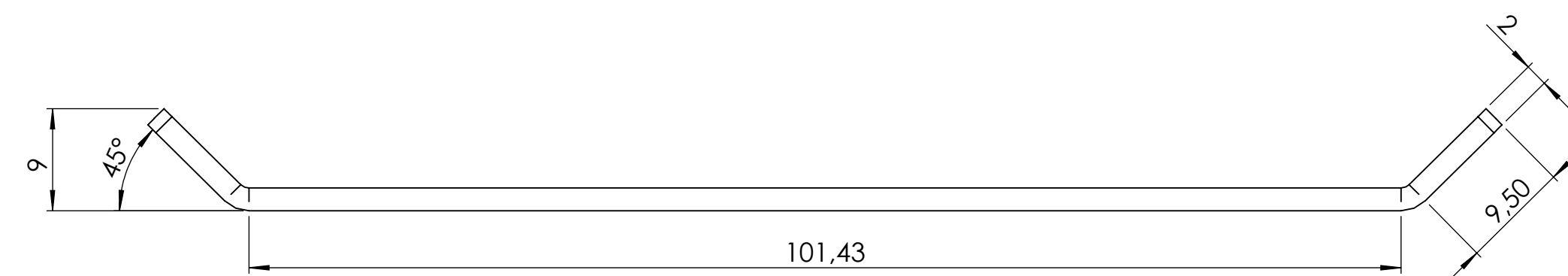
PARTICOLARE SCALA 2:1
